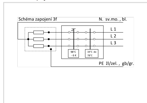
Schéma zapojení:
